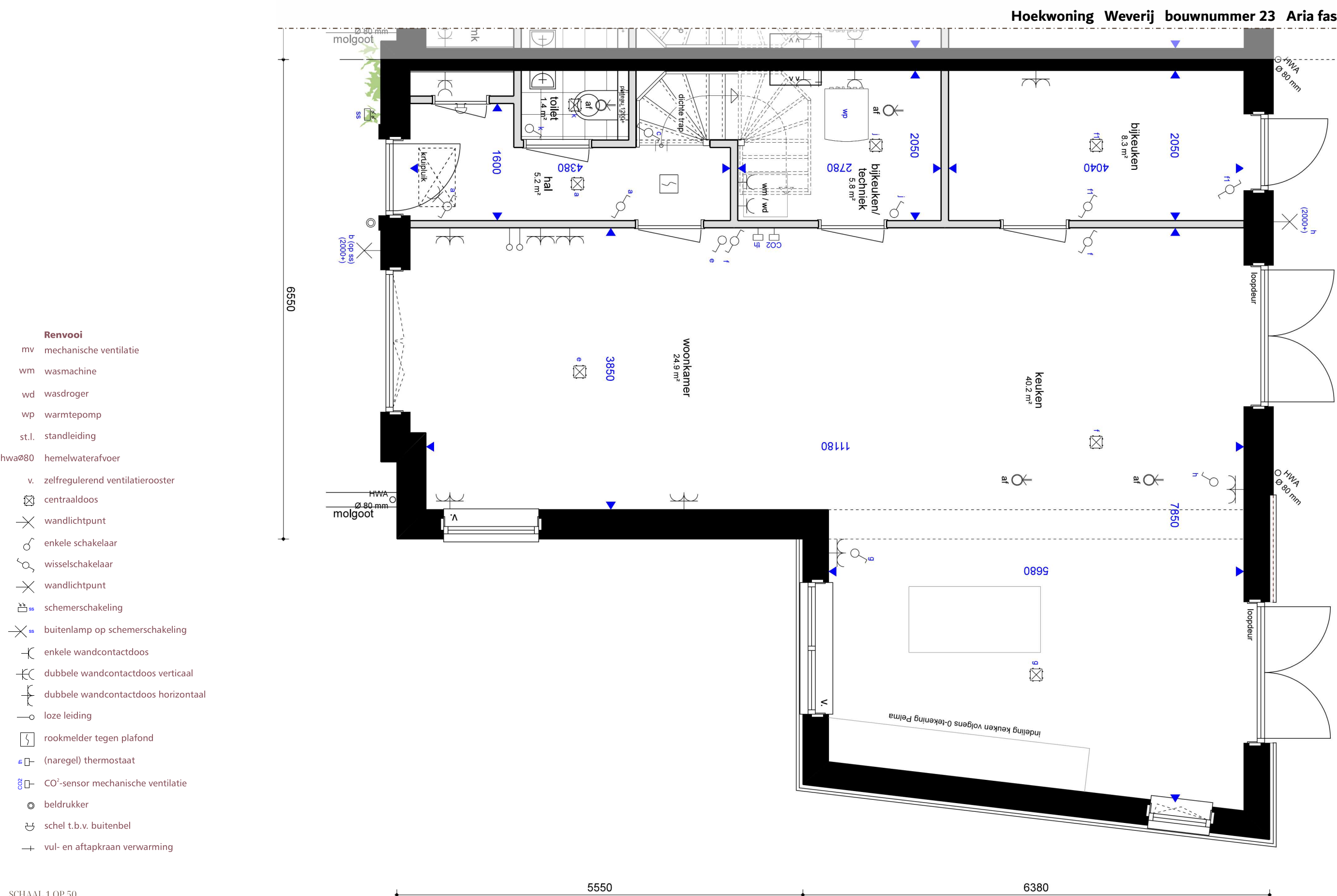
SCHAAL 1 OP 50 Plattegrond ~ Begane grond
